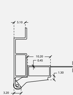
λεπτομέρεια B2 - B2 1:5
