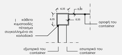
λεπτομέρεια H2 - H2 1:5
