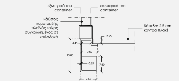
λεπτομέρεια H1 - H1 1:5
