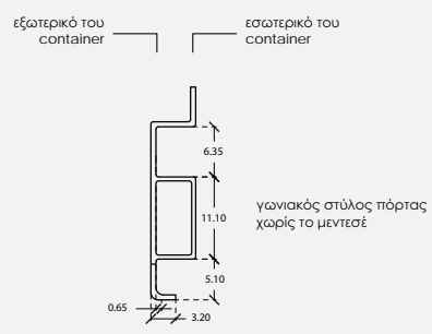
λεπτομέρεια A1 - A1 1:5
